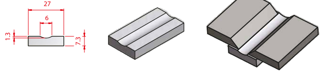
CB 11 - 100
