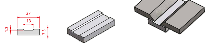
CB 21 - 150
