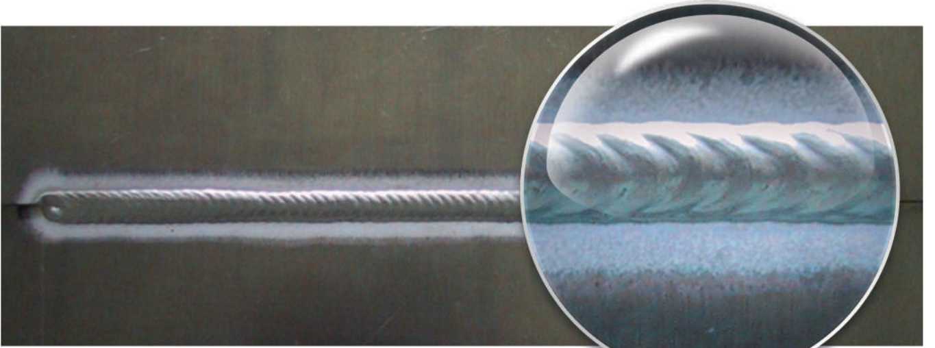
Alüminyum t : 2.0 x 2.0 mm bindirme kaynağı, Kaynak Parametresi : 110A / 40A, Kaynak Hızı: 0.5 m/dk.
