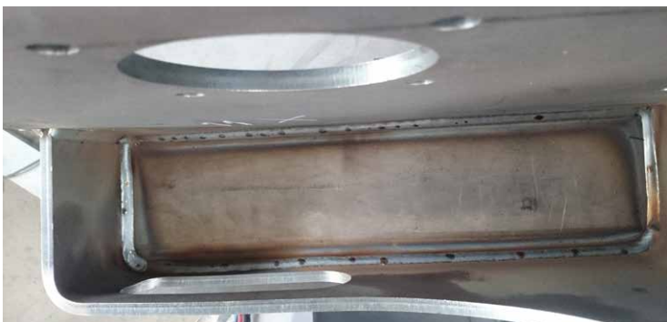
Robotik uygulama sonrasına ait kaynak dikişi görselleri.
