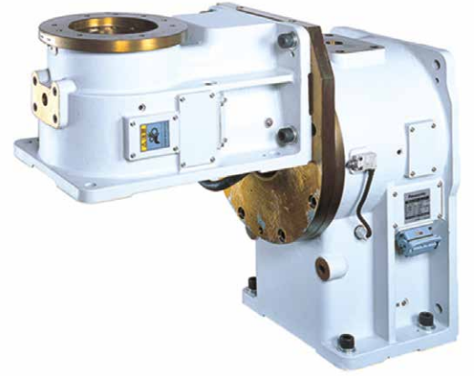
500 Kg.'lık pozisyonerin 1000 Kg.'lık pozisyonere montajı ile elde edilen iki eksenli pozisyoner örneğidir.
