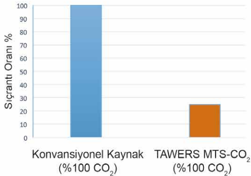
%100 CO 2 ile MAG Kaynağı
