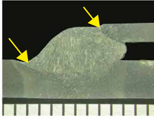
Pulse - MAG Kaynağı 26,8 V (Malzeme: St 37)
